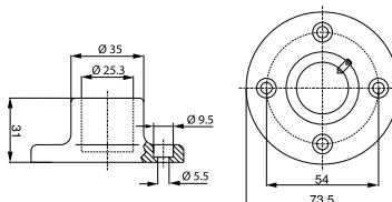
Схема сверления отверстий для сигнальных маяков КSB
