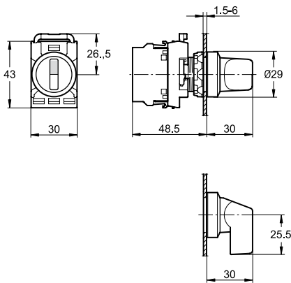
Переключатель
