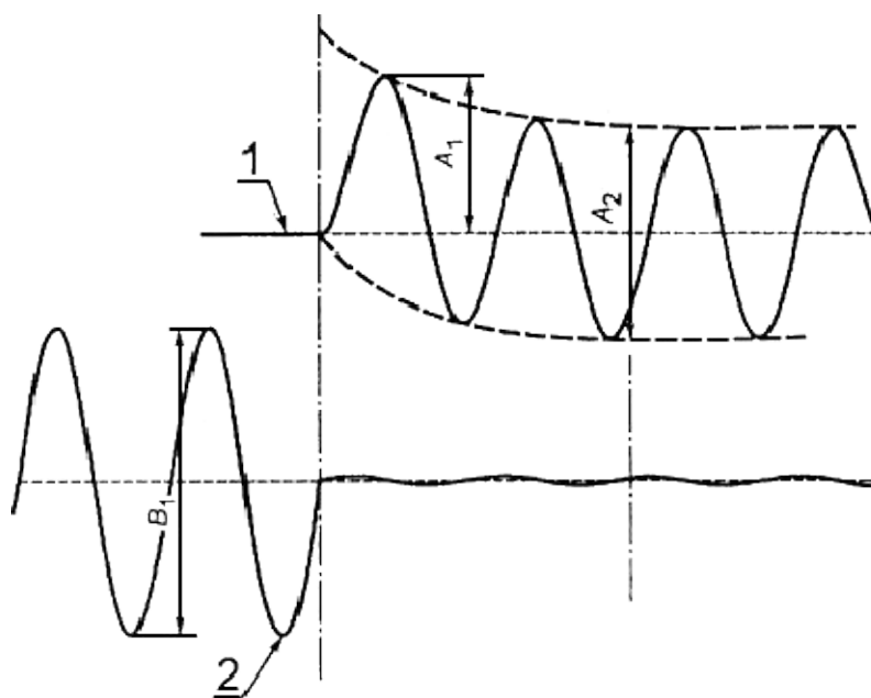
1 - напряжение; 2 - ток
