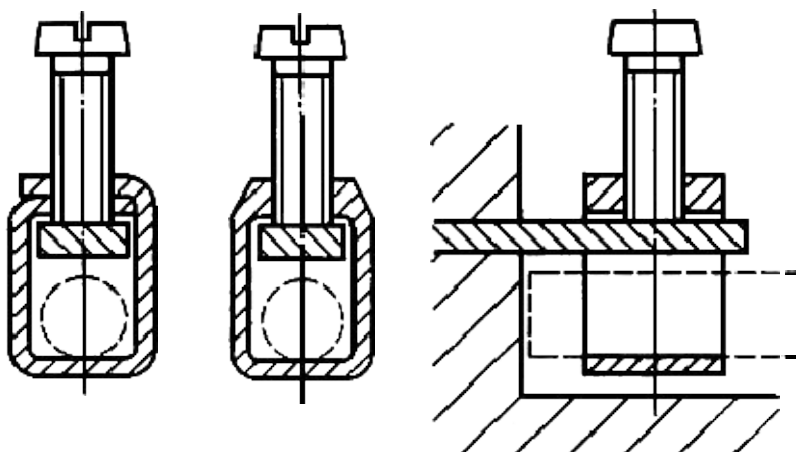
Выводы с хомутиком
