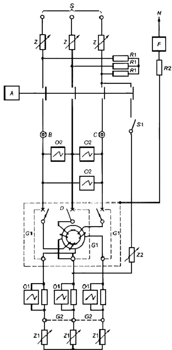
Рисунок 7 - Испытательная цепь для проверки номинальной наибольшей коммутационной способности трехполюсного АВДТ в трехфазной сети (9.12)
